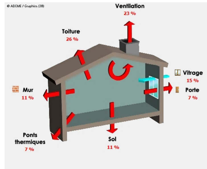
Répartition des pertes de chaleur du logement.
